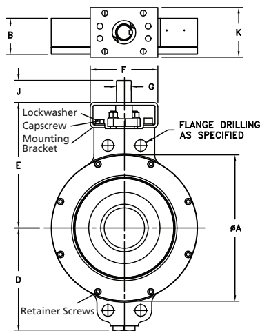
S42 - Wafer / S43 - Lug
